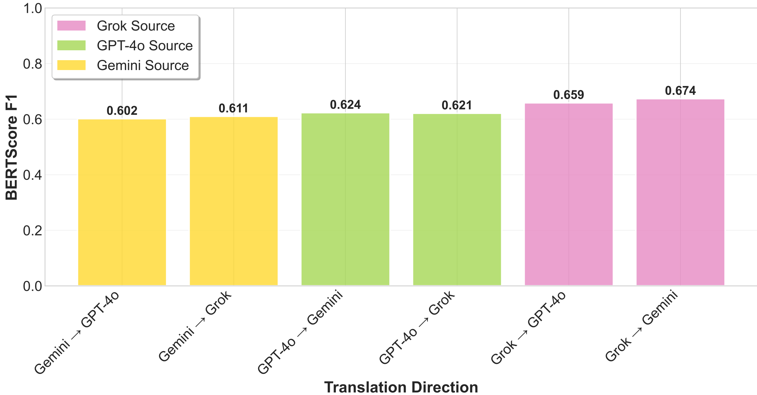
BERTScore F1 Performance
